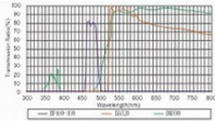
B激發光波濾色組件 Blue Excitation
